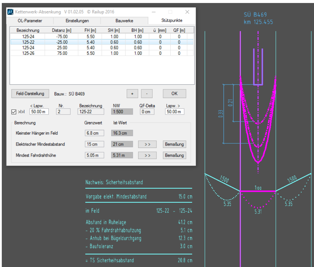
Modul Kettenwerksabsenkung
